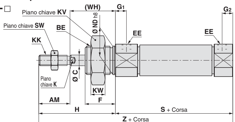
Filettatura anteriore/Base
