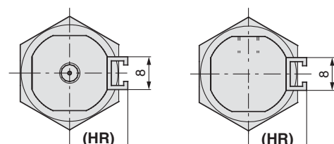
Attacco assiale su testata posteriore
