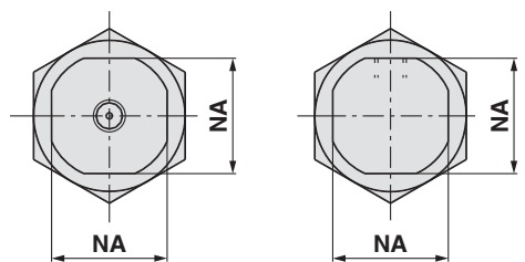
Attacco assiale su testata posteriore
